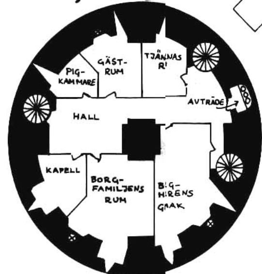
Tredje våningen
